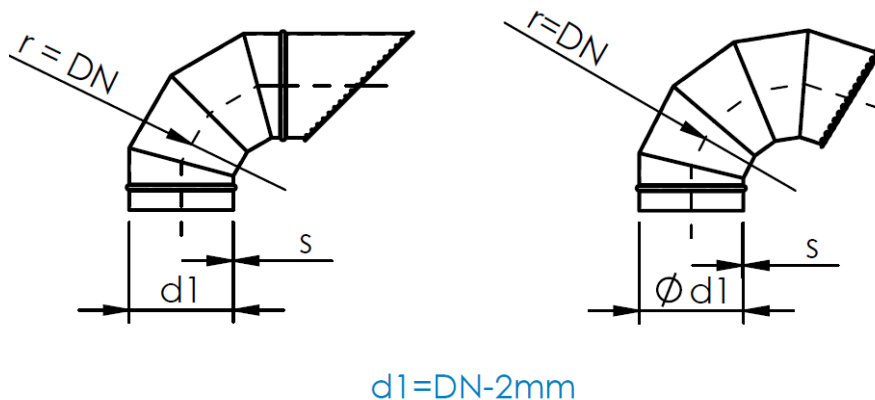
strešni izpihovalni kos z mrežo SIA-90° fi DN SIA-120° fi DN
